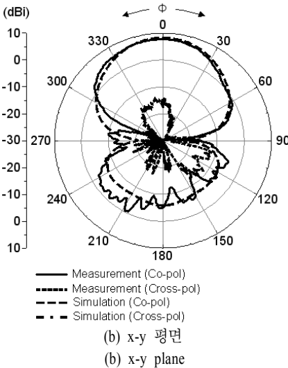
그림 11. 5.7 GHz에서의 복사 패턴 Fig. 11. Radiation patterns at 5.7 GHz.
