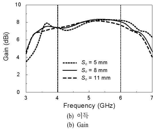
그림 5. Driver와 reflector 사이 간격에 따른 안테나의 특성 Fig. 5. Characteristic of antenna with respect to the distance between driver and reflector.
