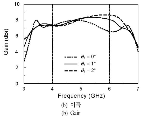
그림 6. 테이퍼된 각도( \theta_1 )에 따른 안테나의 특성 Fig. 6. Characteristic of antenna with respect to the tapered angle( \theta_1 ).
