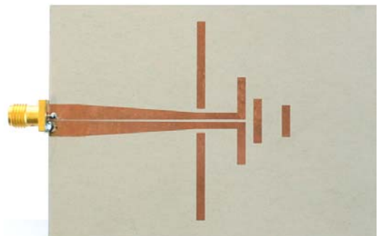
그림 7. 제작된 Yagi-Uda 안테나 Fig. 7. Photograph of the fabricated Yagi-Uda antenna.
